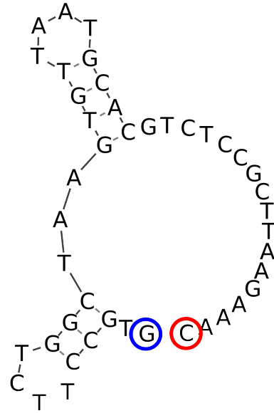
ND6-ND3 IGR
