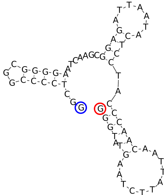
COIII-ATP6 IGR
