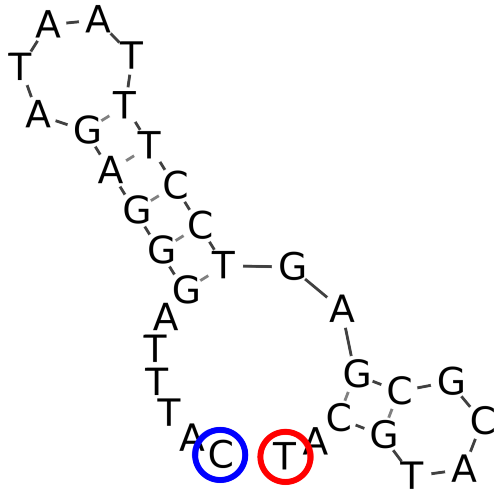
ND1-CytB IGR
